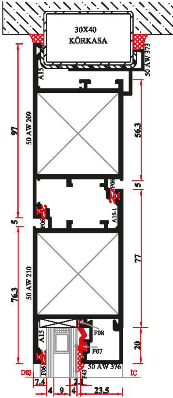
ÖLÇEK:1/2 2 NOLU DETAY
